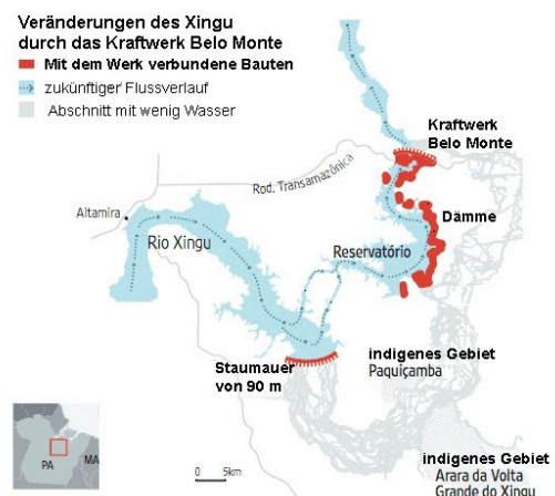
Darstellung des veränderten Flussverlaufes des Xingu und der notwendigen Baumaßnahmen zur Errichtung von ‚Belo Monte‘
