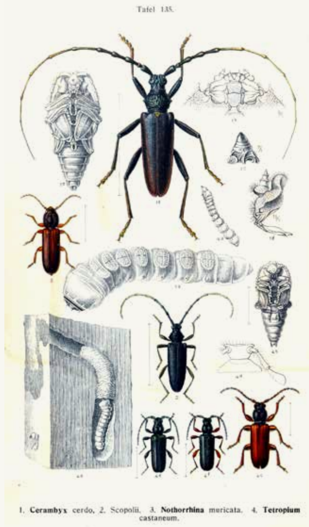
Abb. 15: Käfer und Larve des Heldbocks; Quelle: Reitter 1912
