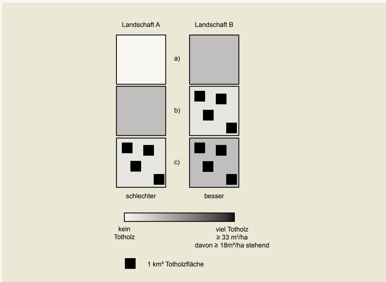
Abb. 5: Grundsätze für die Verteilung von Totholz innerhalb einer Waldlandschaft (Bütler & Schlaepfer 2004)
