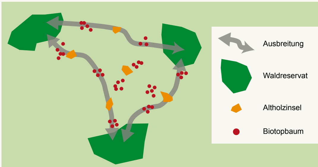
Abb. 6: Lebensraumverbund von Waldreservaten, Altholzinseln und Biotopbäumen (Lachat & Bütler 2007)
