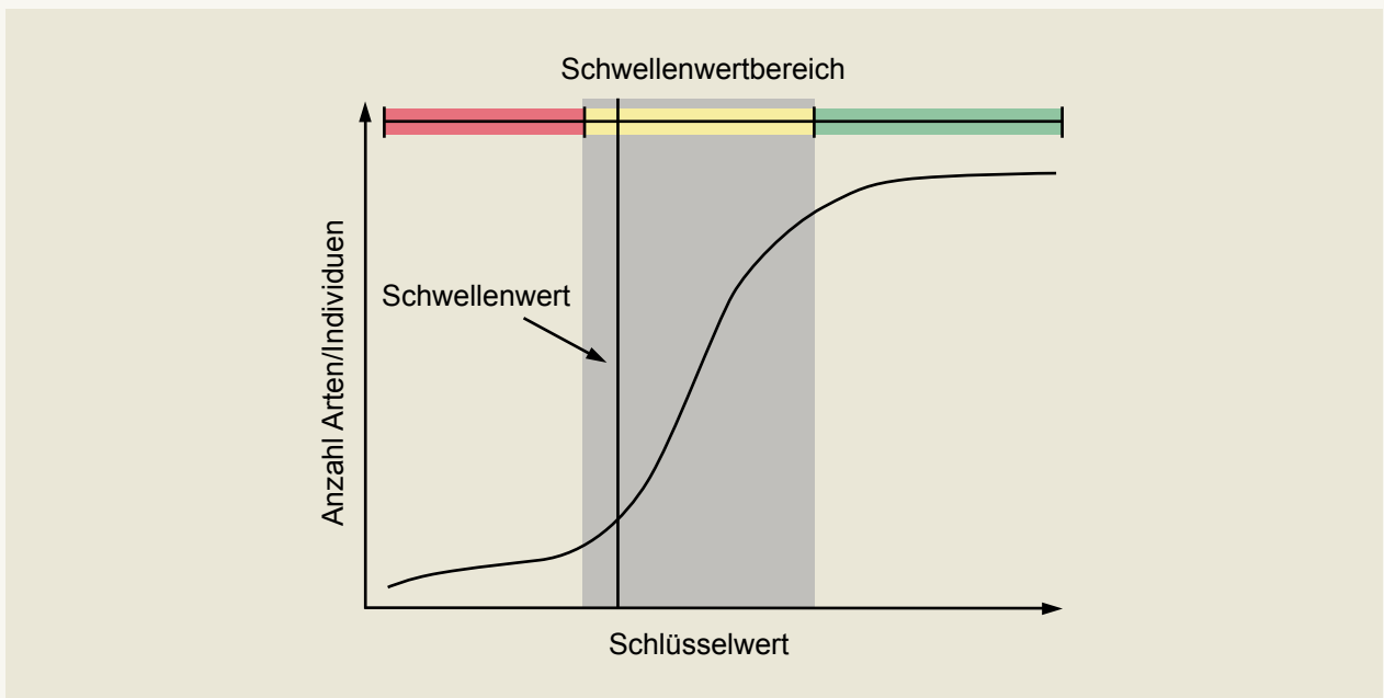
Abb. 2: Schlüssel- und Schwellenwerte (Moning 2013)
