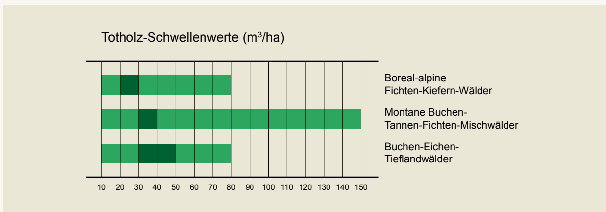
Abb. 3: Totholz-Schwellenwerte für verschiedene xylobionte Arten in europäischen Wäldern (dunkler Bereich), heller Bereich: Bandbreite, in dem die untersuchten Arten vorkommen (Müller & Bütler 2010)
