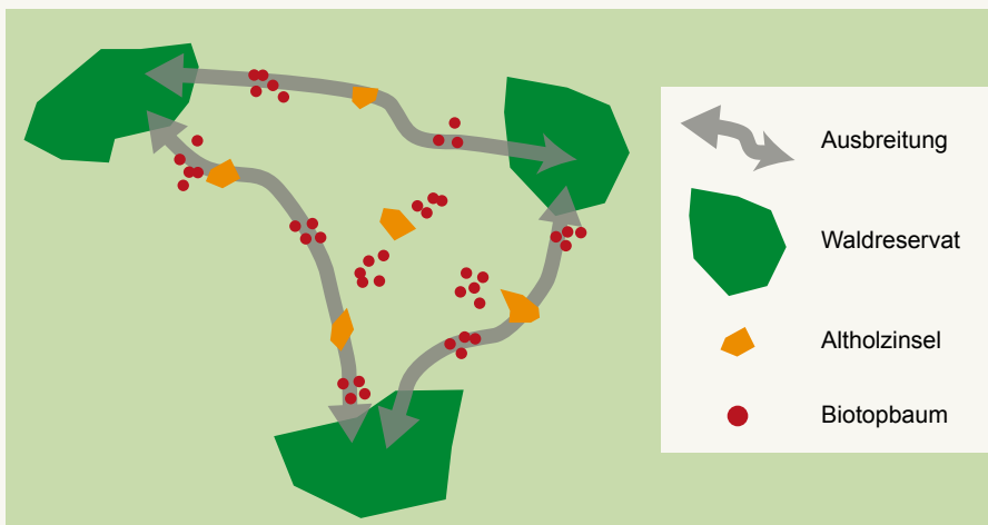
Abb. 25: Darstellung der Vernetzung der Elemente (verändert nach Lachat & Bütler 2008)
