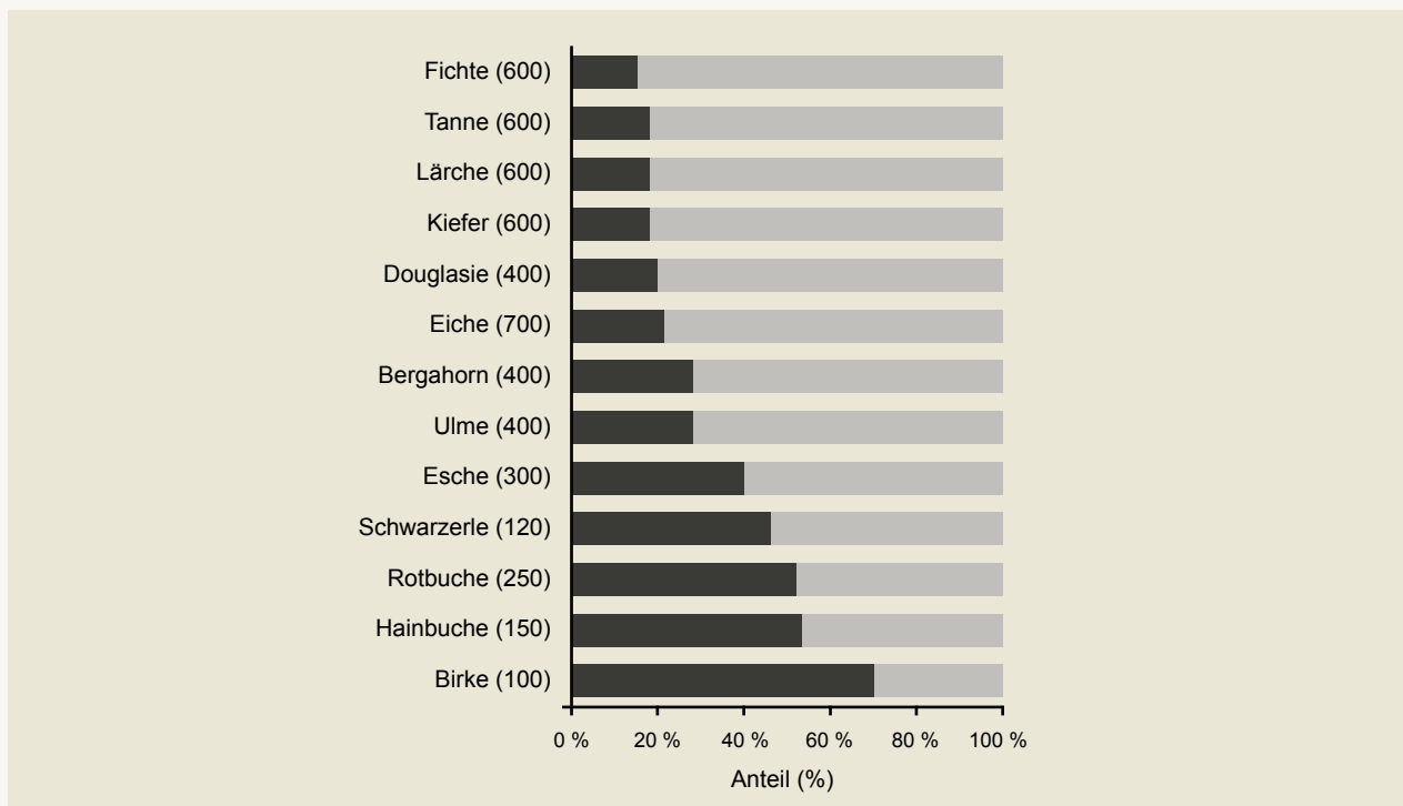
Abb. 4: Anteil des durchschnittlichen Umtriebsalters (schwarz) am natürlichen Lebensalter verschiedener Baumarten. Der graue Bereich fehlt üblicherweise im Wirtschaftswald (Jedicke 2008).
